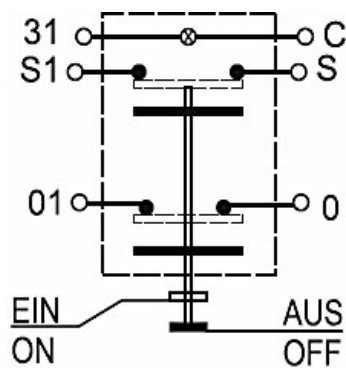
Schaltbild
