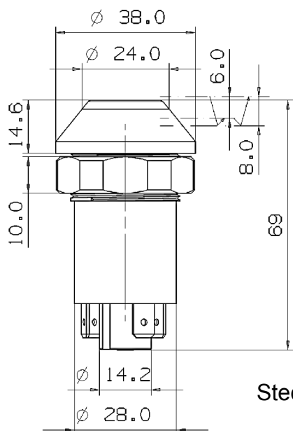
Stecker Anordnung
